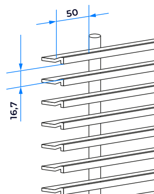
GL-B15
