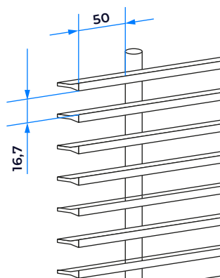
GL-B0
